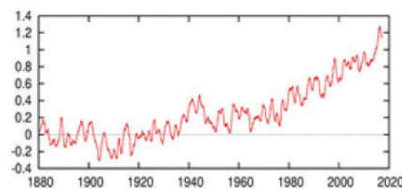
Wereldgemiddelde temperatuur (GISTEMP, t/m september 2017) ten opzichte van 1880 - 1900 met een 12-maands lopend gemiddelde (Bron: NASA/GISS).
